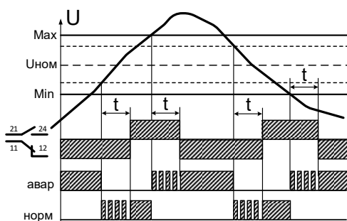
Рис. 2а. Реле напряжения "работа «окном»"
