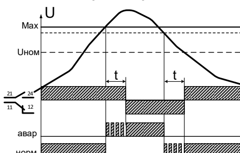
Рис. 2б. Реле максимального напряжения "Униз выкл"
